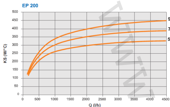
Dolní trubkový výměník
